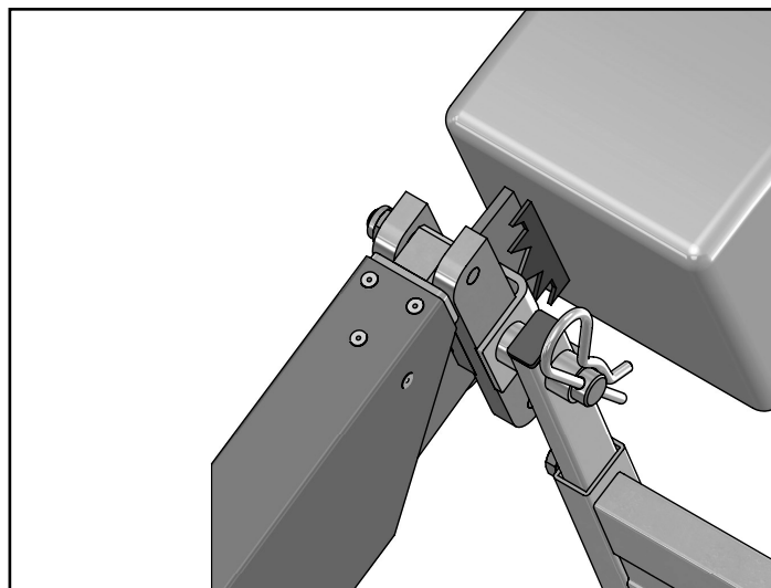
Dispositif de serrage avec tronçonneuse
